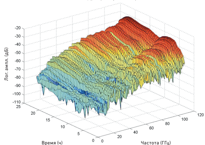
Дрейф модуля вектора S11
