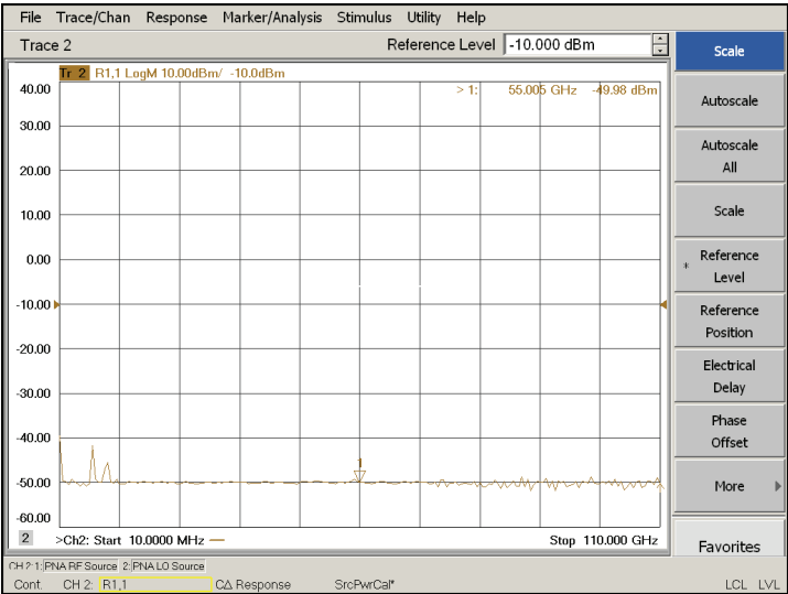
Рис. 2: Наименьший уровень выходной мощности, равный 50 дБм в диапазоне от 10 МГц до 110 ГГц
